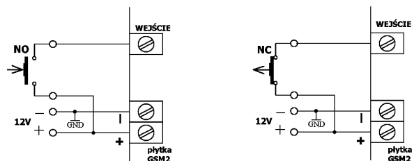
A. Sterowanie przez podanie +12V Ustawić poziom aktywny H
