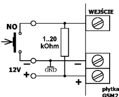
C. Sterowanie przez podanie masy Ustawić poziom aktywny L
